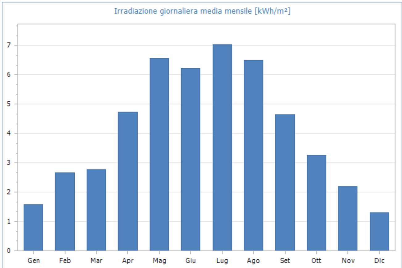
Fig. 1: Irradiazione giornaliera media mensile sul piano orizzontale [kWh/m 2 ]- Fonte dati: UNI 10349:2016 - Stazione di rilevazione: Airola
